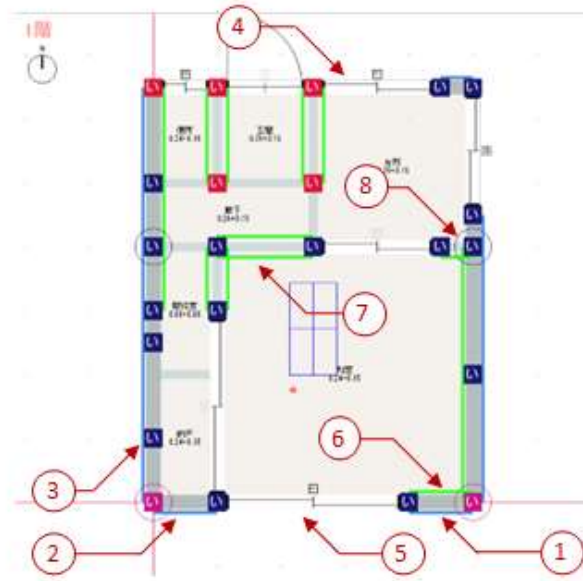
1階平面図
